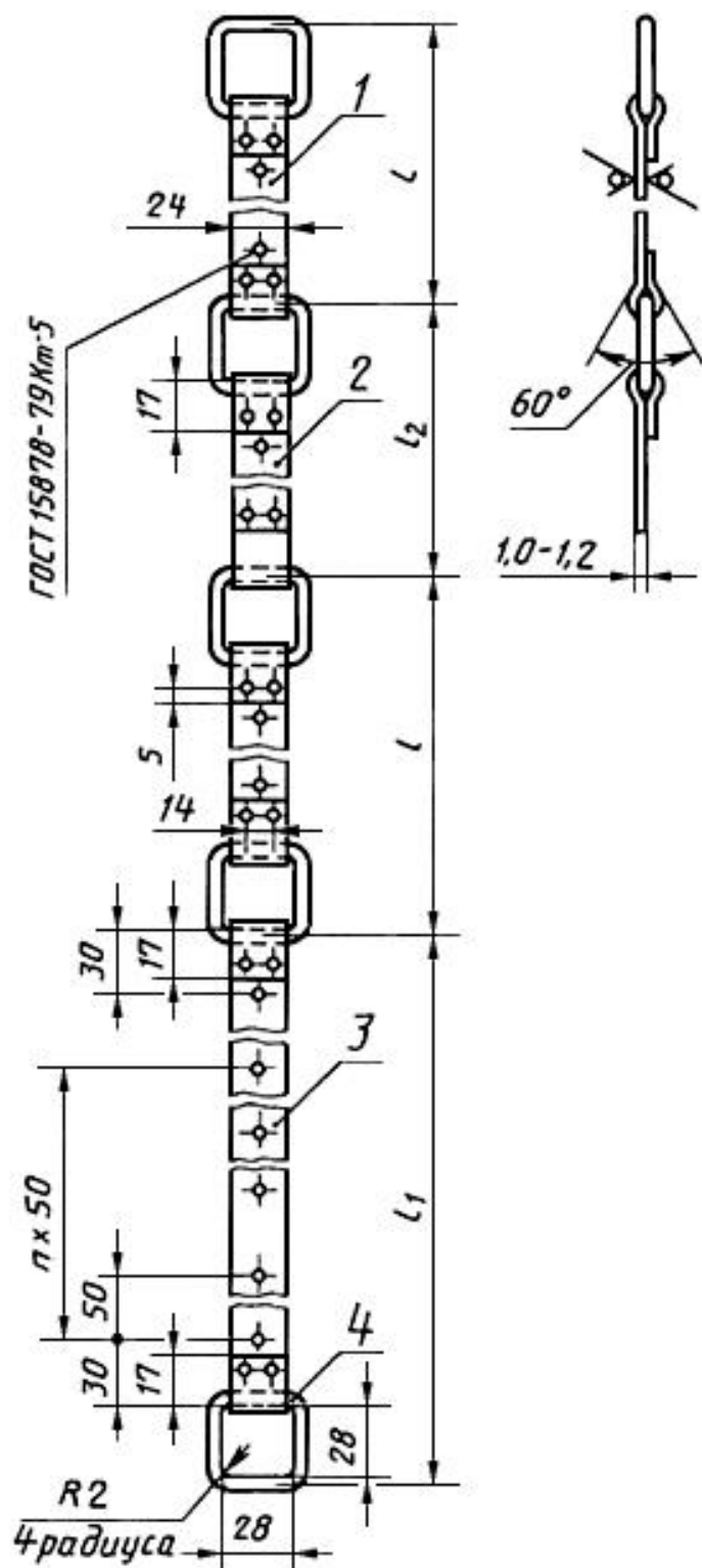
Черт.20. Металлические пояса для ящиков типа VI
